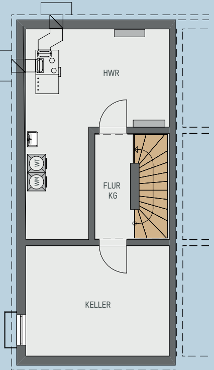
KELLERGESCHOSS
