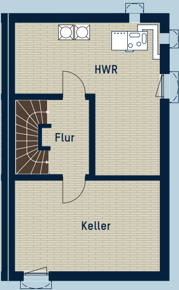
KELLERGESCHOSS
